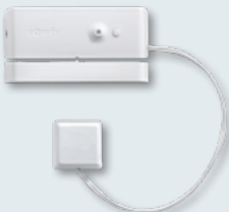
Somfy Funk-Öffnungs- und Glasbruchmelder detektiert das Öffnen von Fenstern und das Einschlagen der Fensterscheibe.
